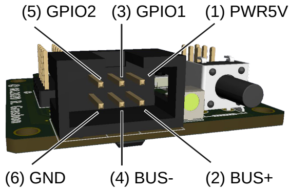
Pinbelegung H3
