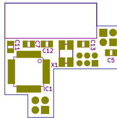
Unterseite
