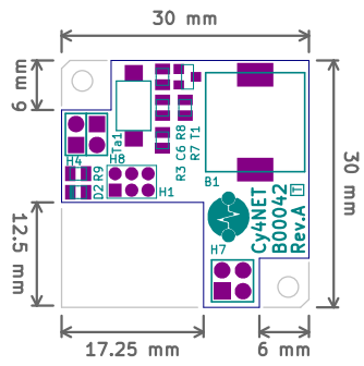
Oberseite
